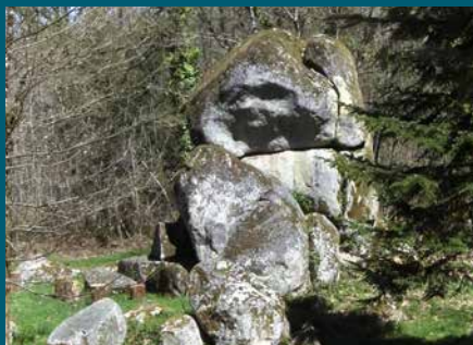
Chaos granitique de Roche Eisode
